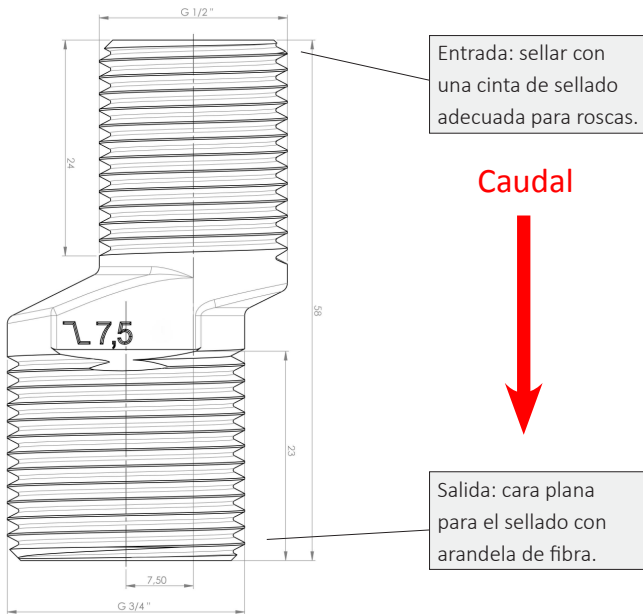
Imagen: HL2024 Connect-S con excentricidad de 7,5 mm (dimensiones en mm).
