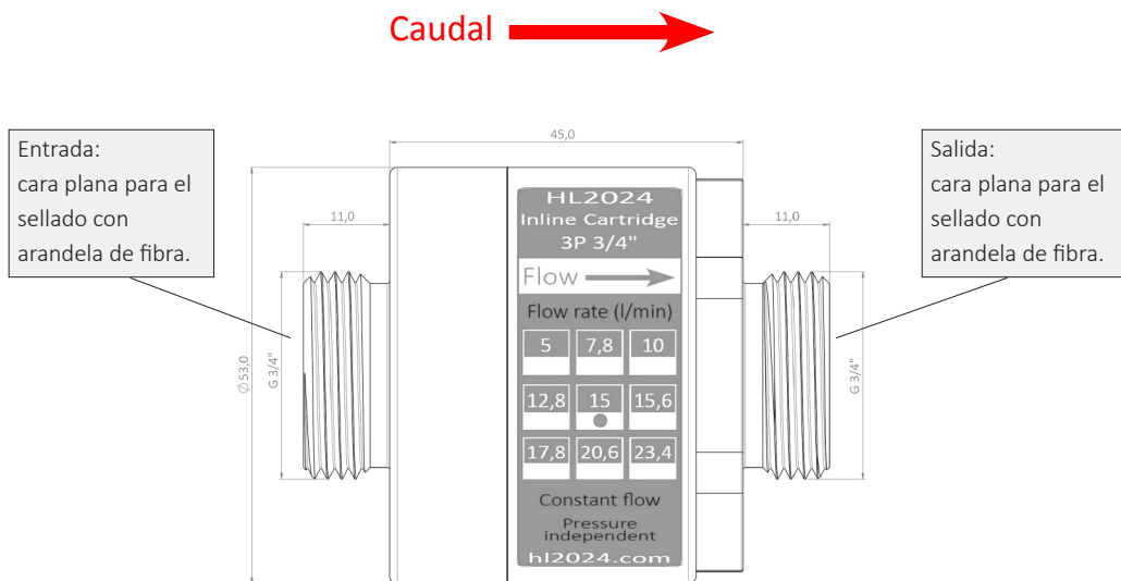
Imagen: HL2024 Inline Cartridge 3P 3/4" (dimensiones en mm)
