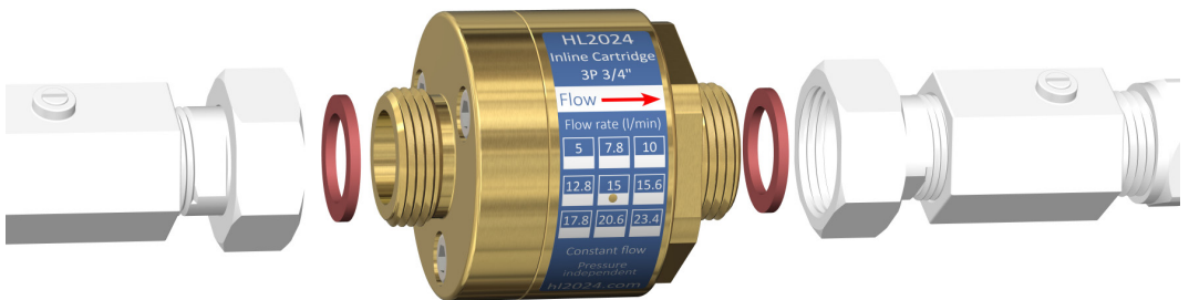
Imagen: HL2024 Inline Cartridge 3P 3/4" montado en la tubería
